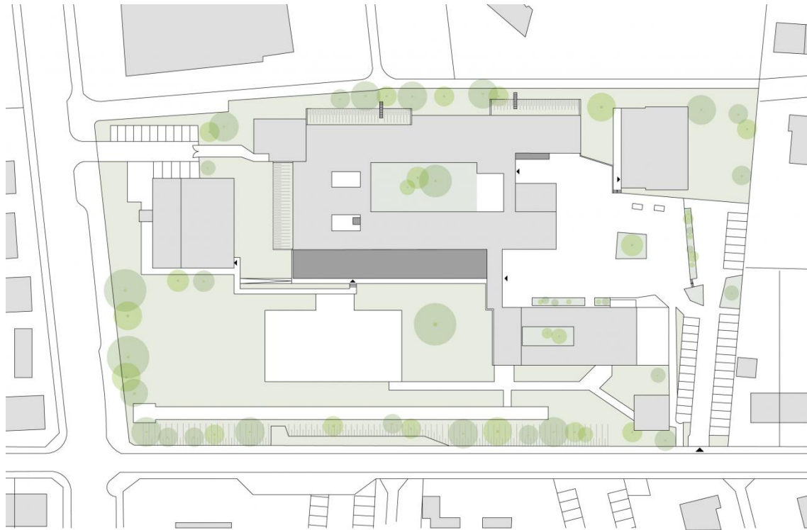
Lageplan
